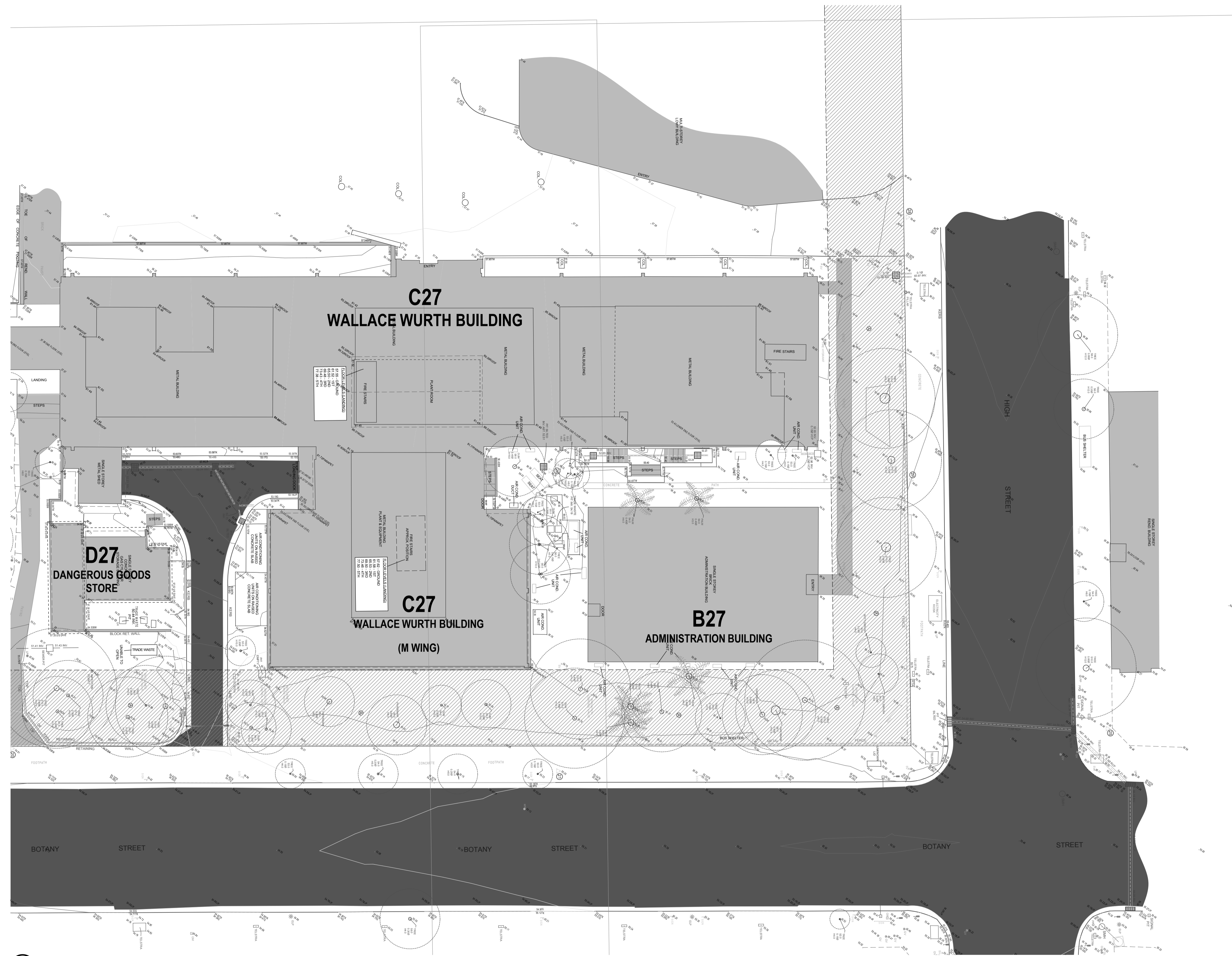
1 SURVEY 100222 1:200
