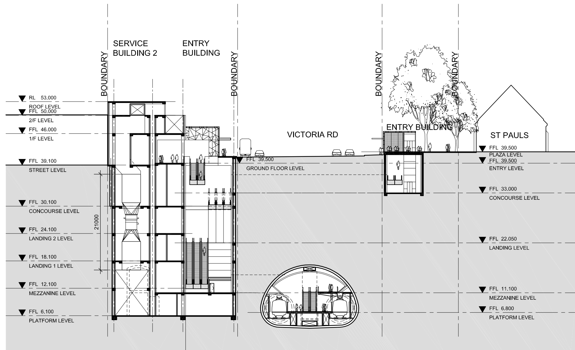
01 SECTION A-A 1:500
