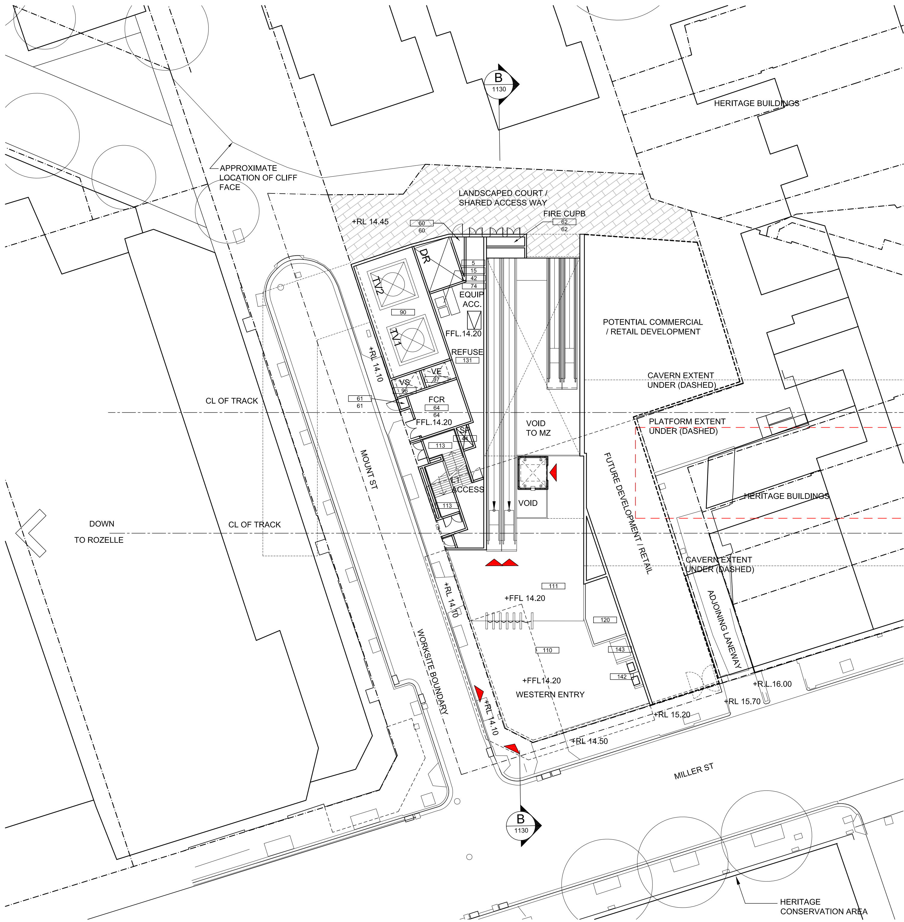
01 STREET ENTRY LEVEL PLAN - FFL 14.20 nom
