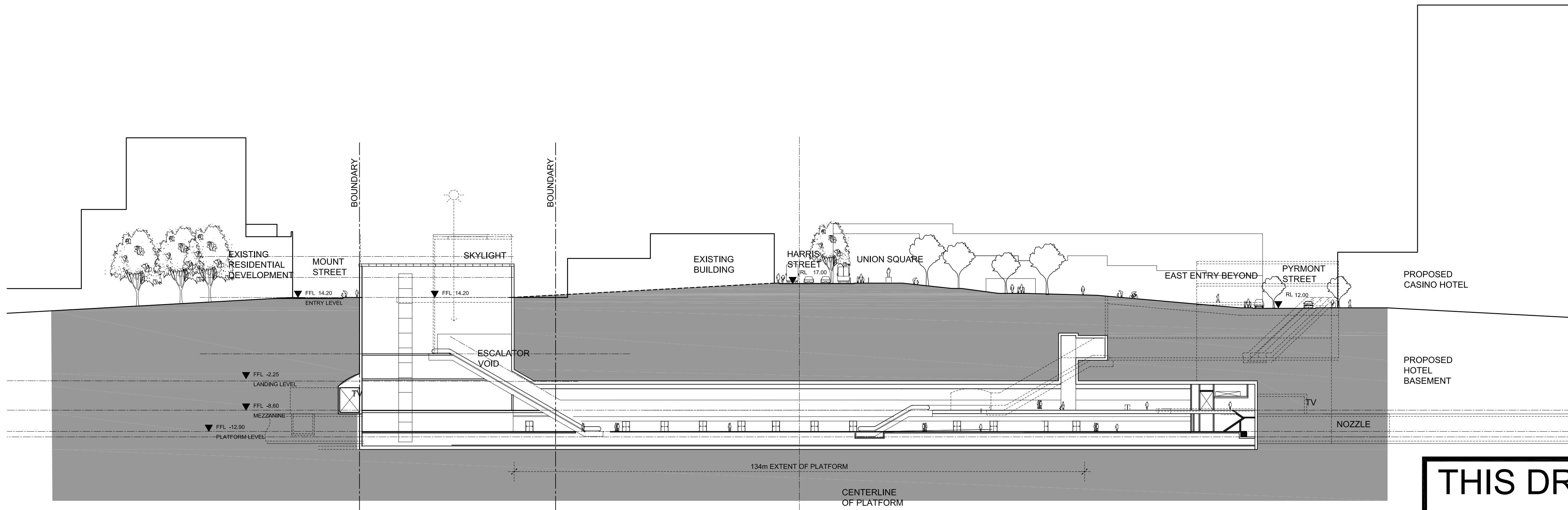
CC LONG SECTION 0200
