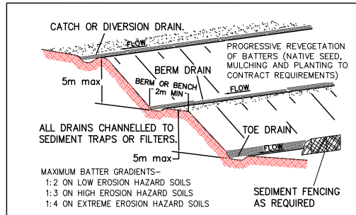
BATTER STABILISATION
