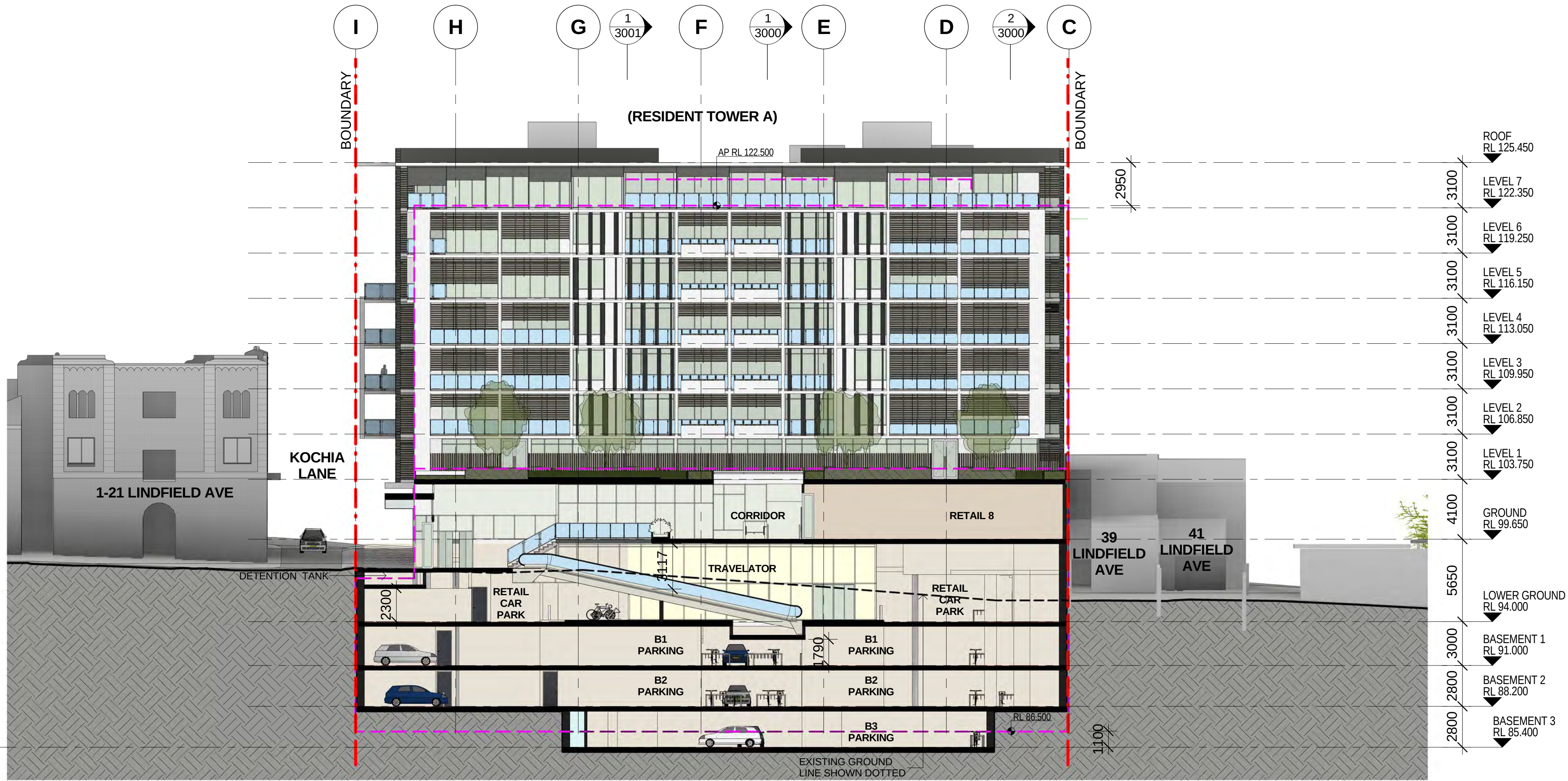
1 SECTION 5 3002 SCALE 1 : 200
