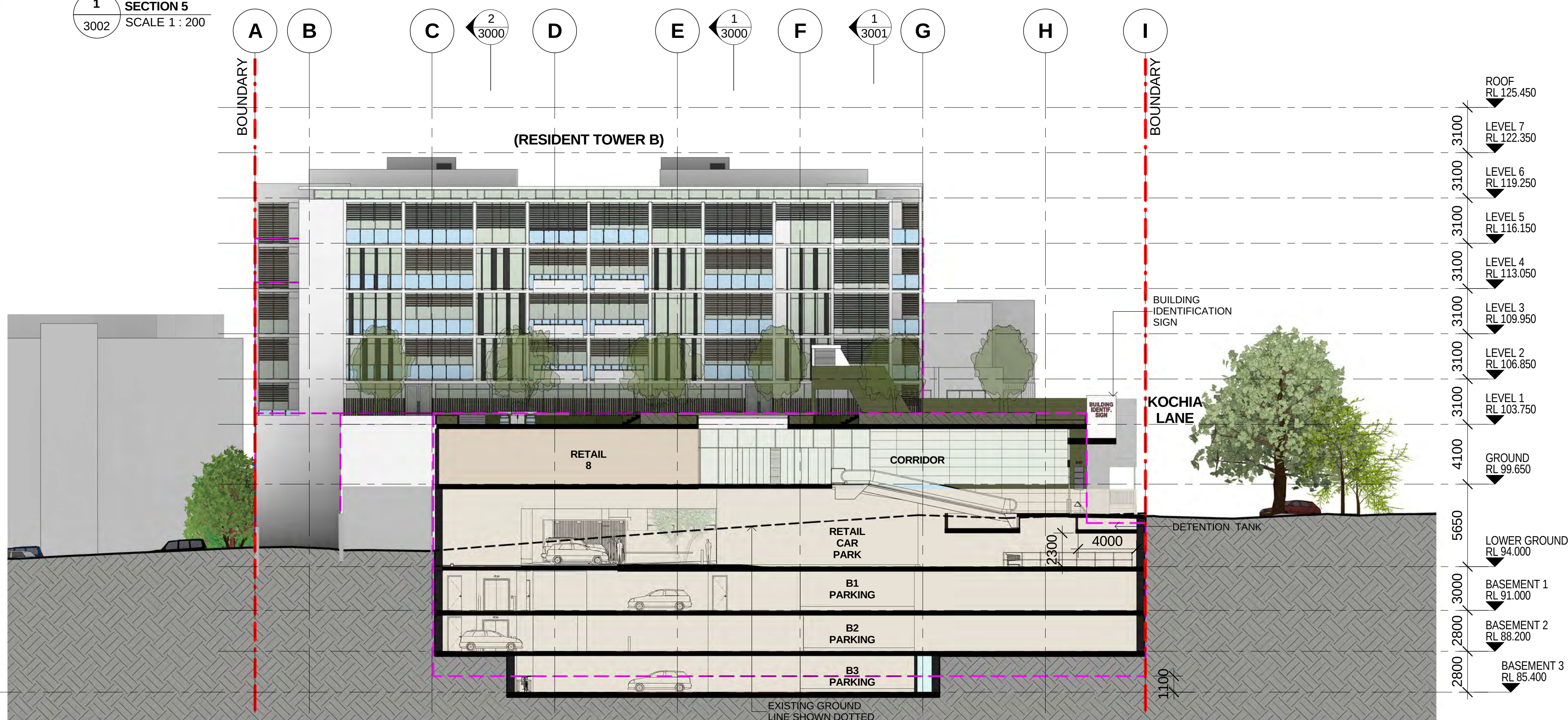
2 SECTION 6 3002 SCALE 1 : 200
