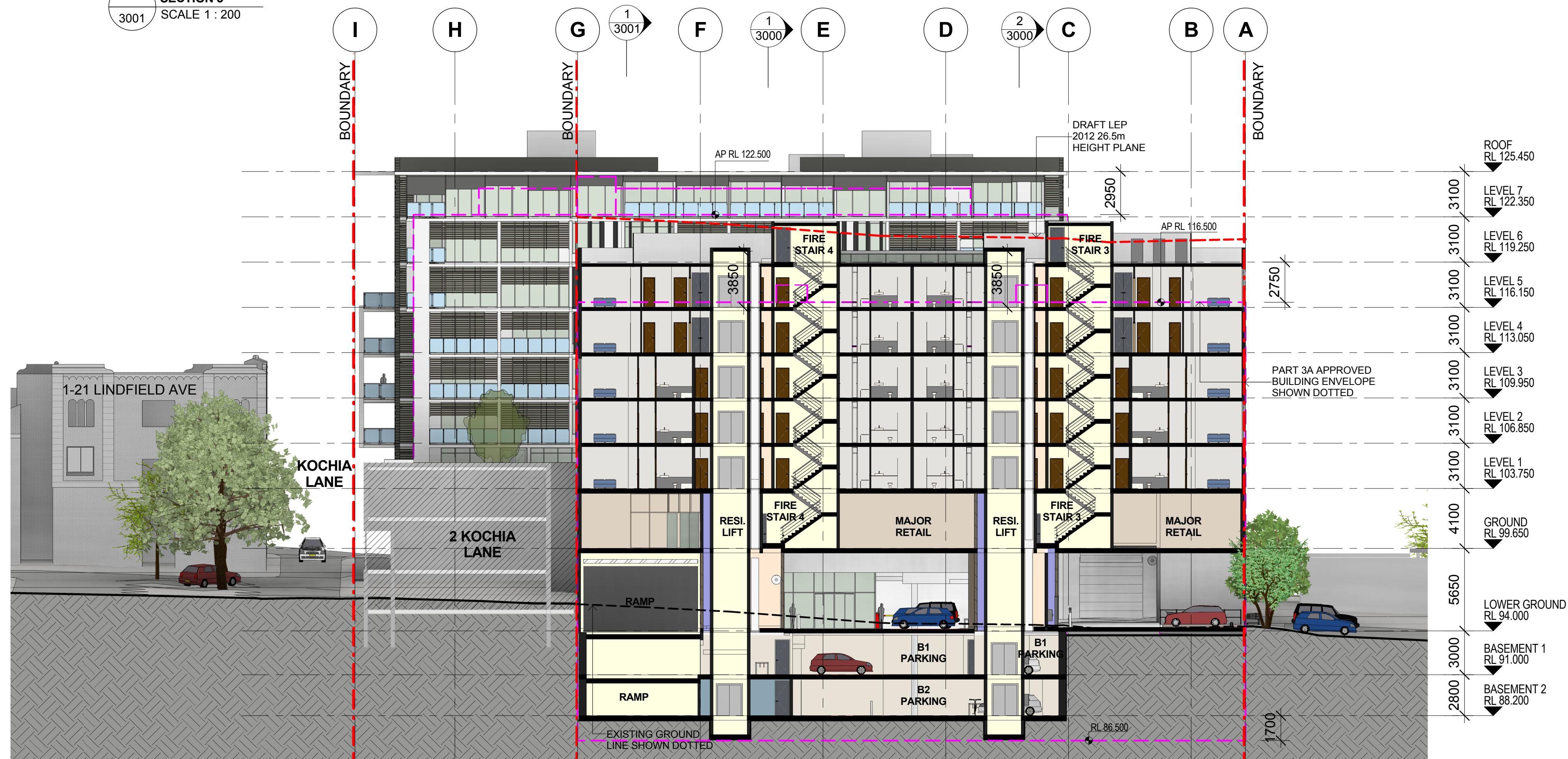
2 SECTION 4 3001 SCALE 1 : 200
