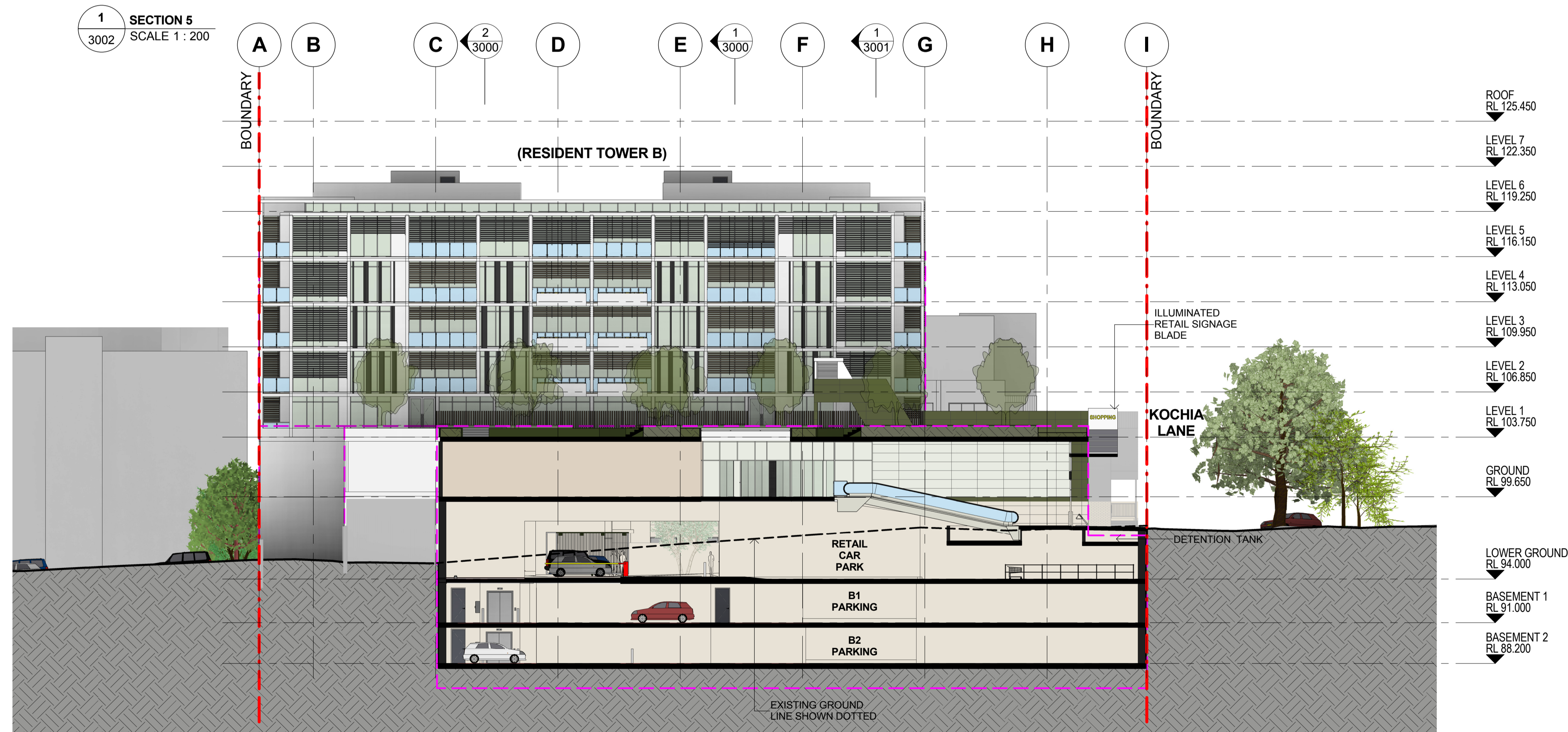
2 SECTION 6 3002 SCALE 1 : 200
