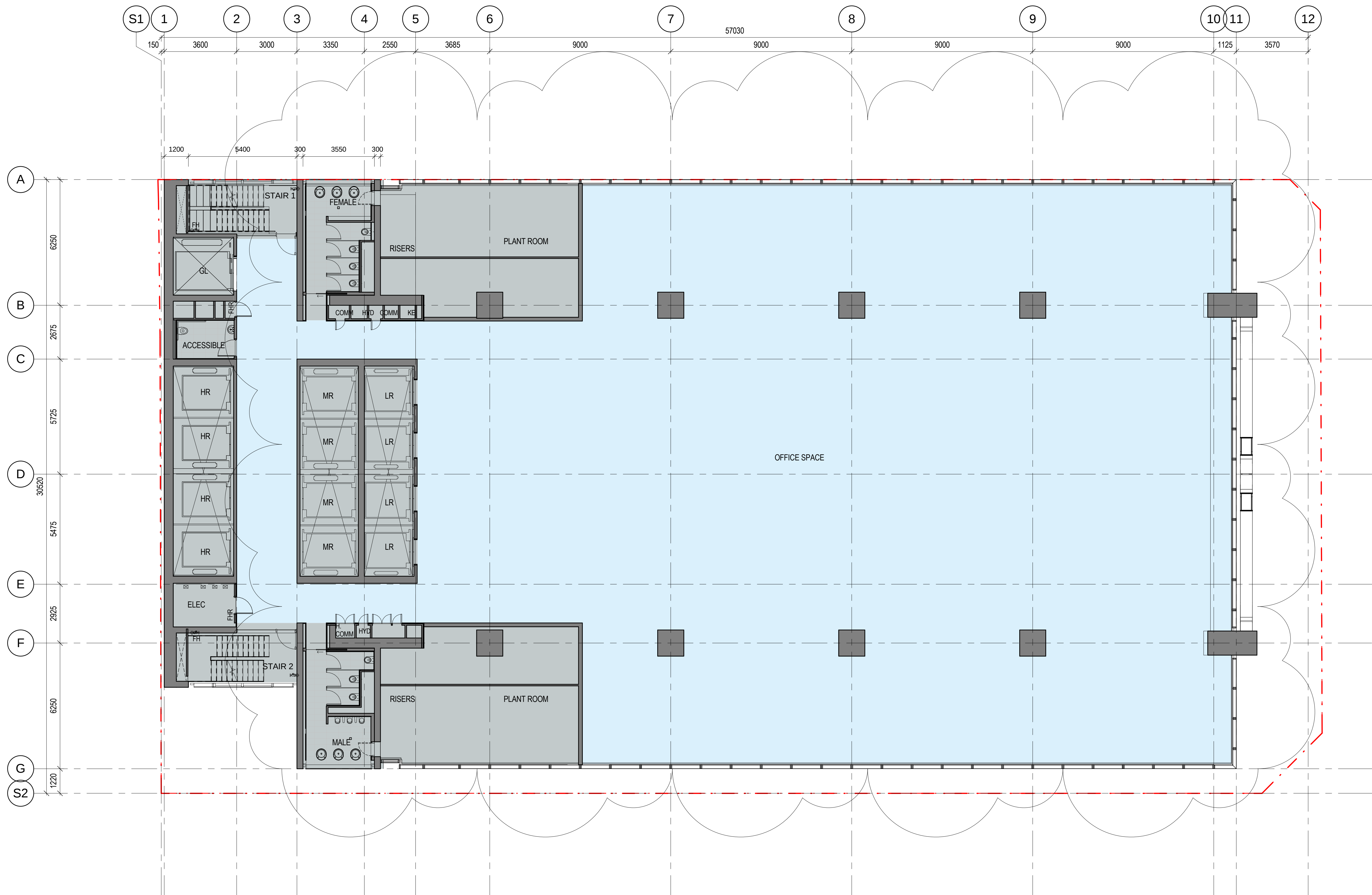
1 Level 2 SCALE: 1 : 100
