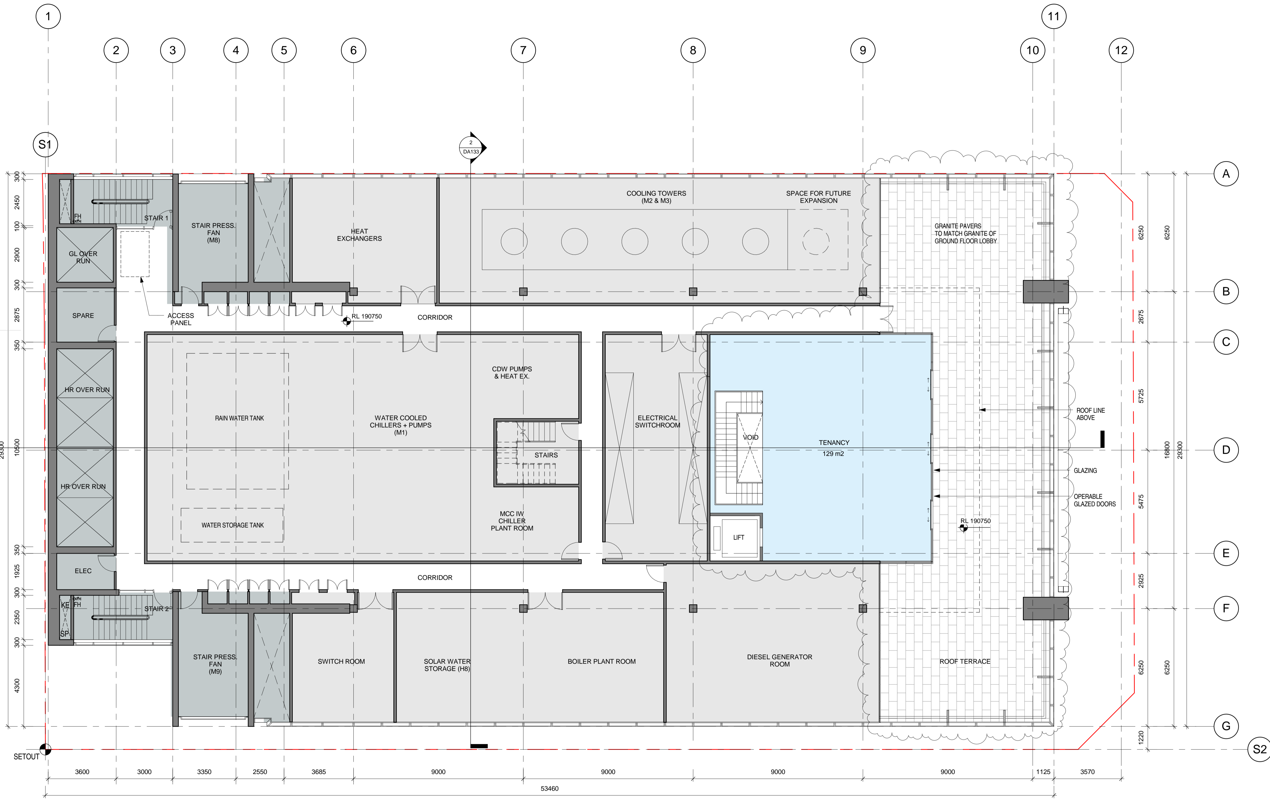
1 Plant Level ARSK-019 Scale: 1:100
