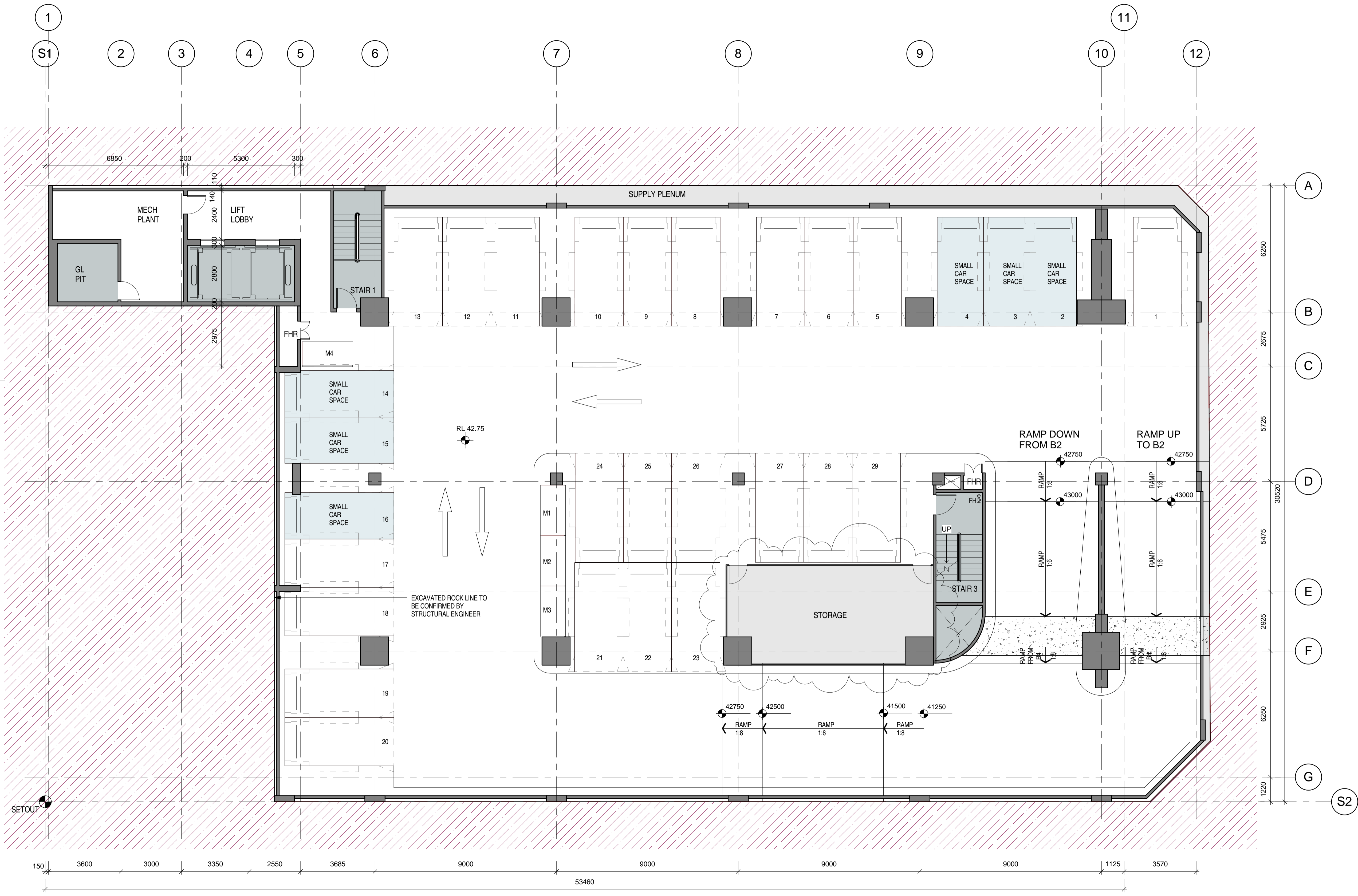
1 Level B3 Plan A2100 Scale: 1 : 100
