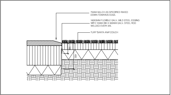
8 STEEL EDGE SECTION 1:10
