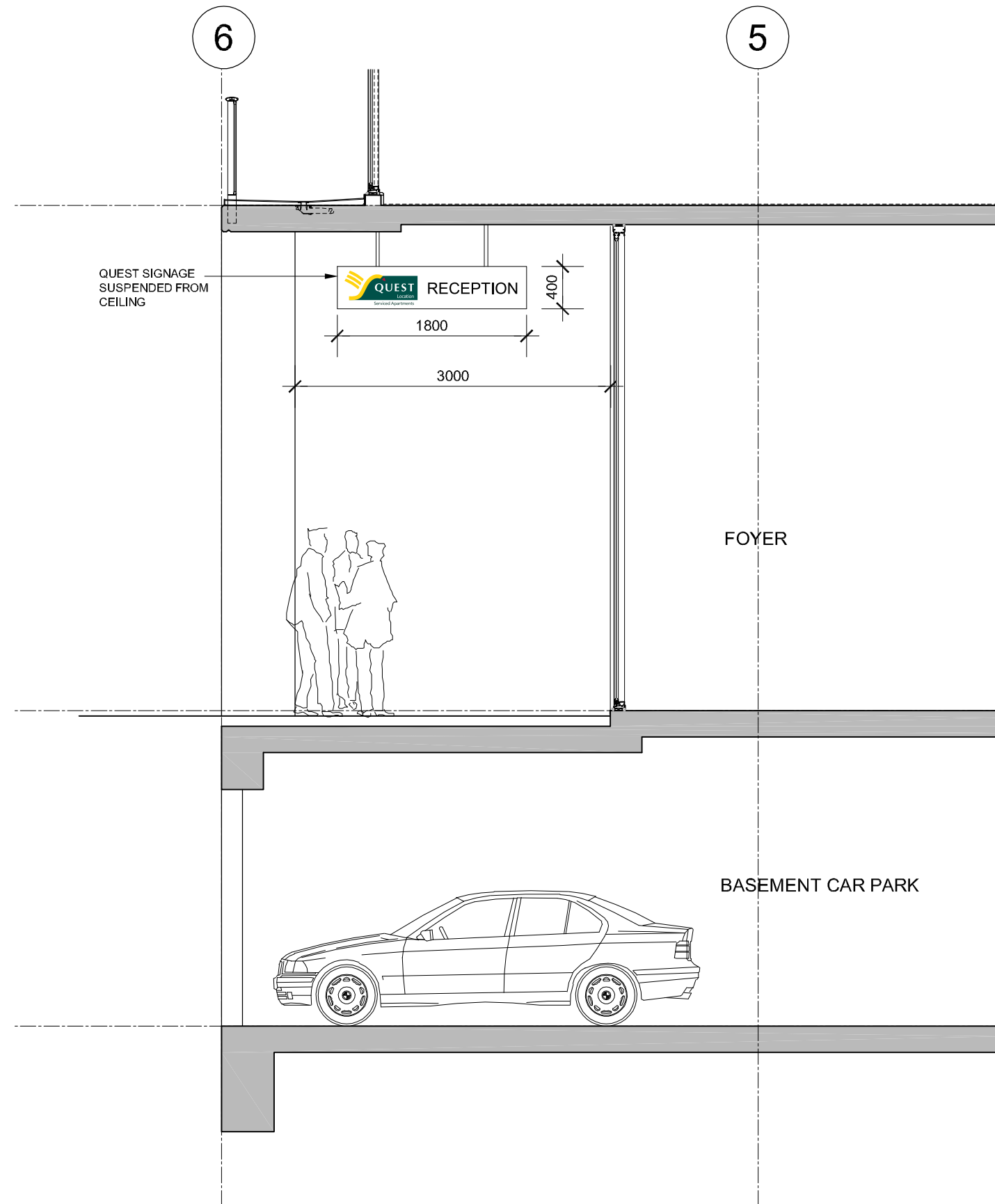
01 FOYER SECTION 1:50
