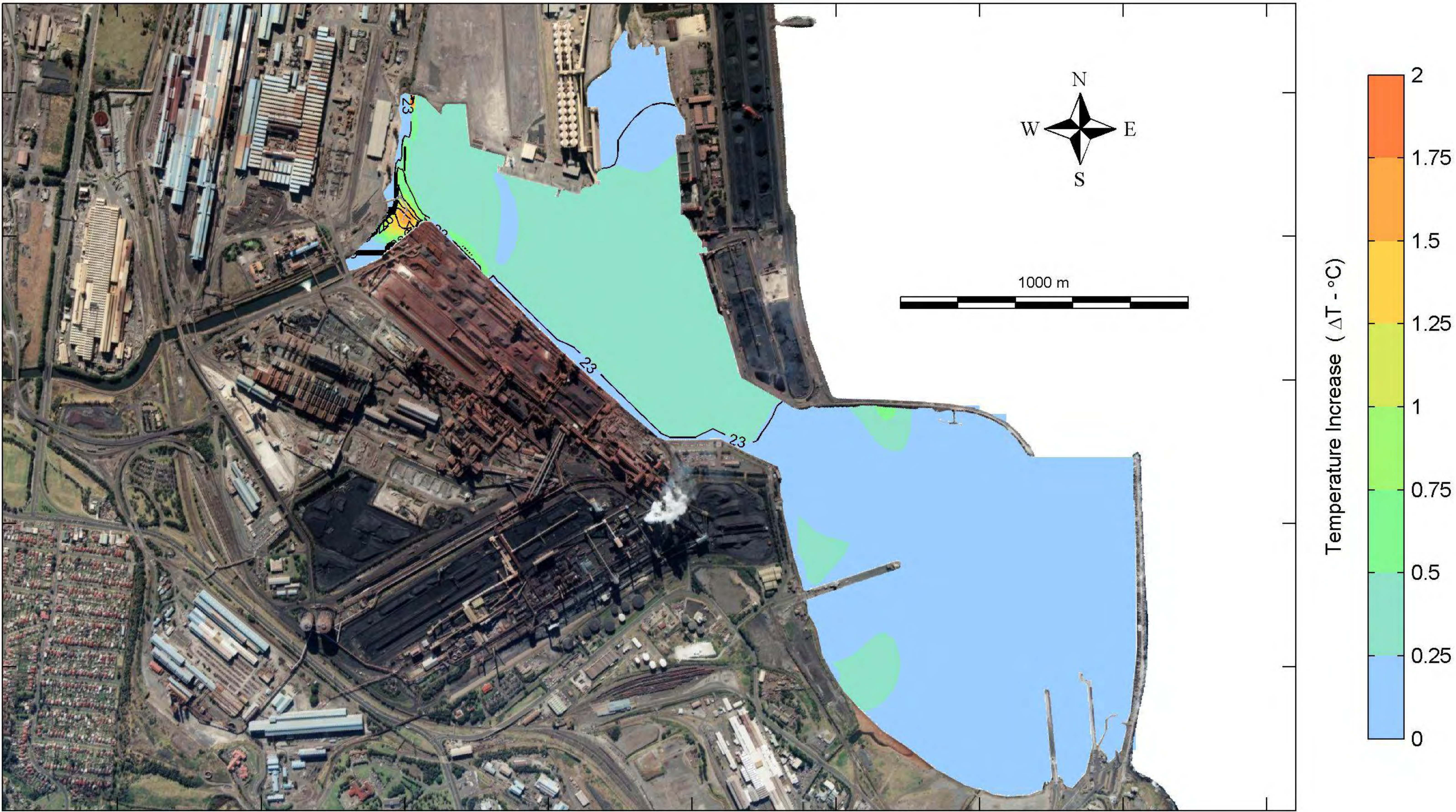
Bottom Layer
