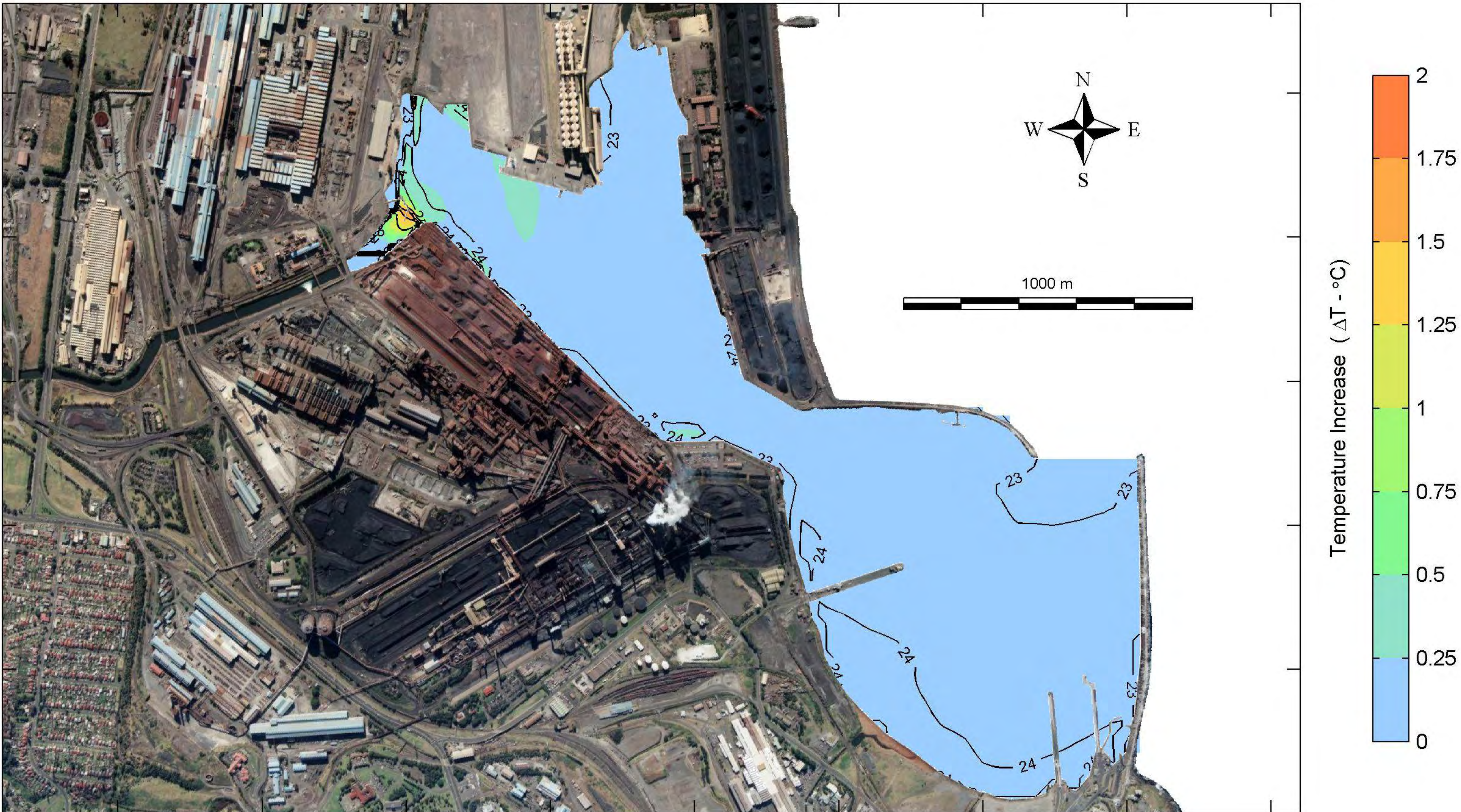
Bottom Layer
