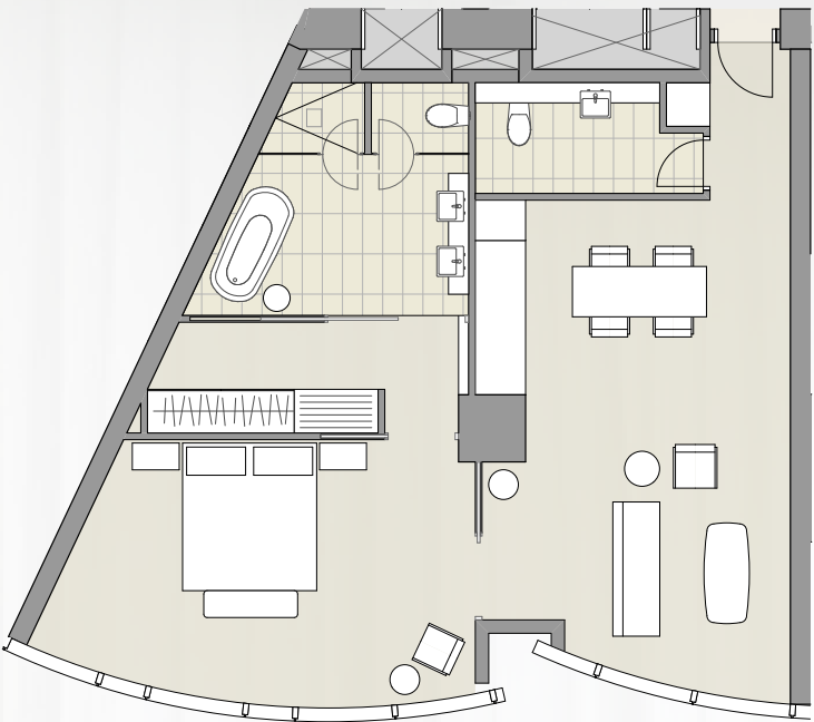
Module D — Centre Suite (double module) — 93sqm NLA — 1:100
