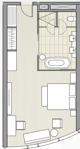
Module B — King or Double Queen — 45sqm NLA — 1:100
