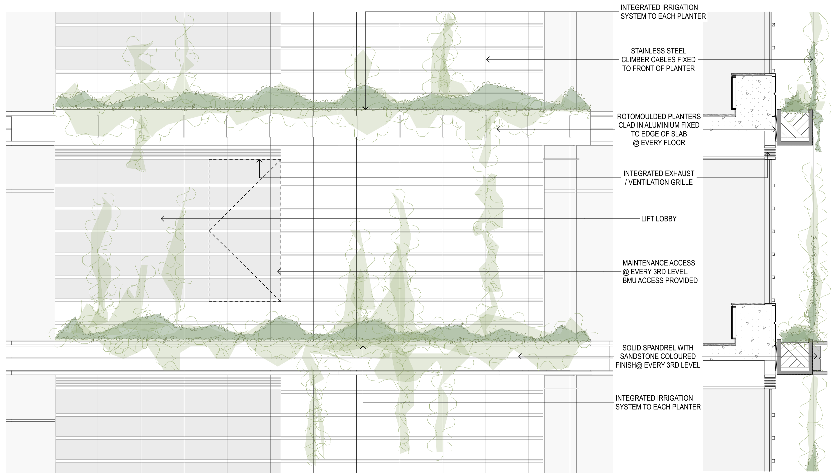
1 ELEVATION Elevation 1:25
