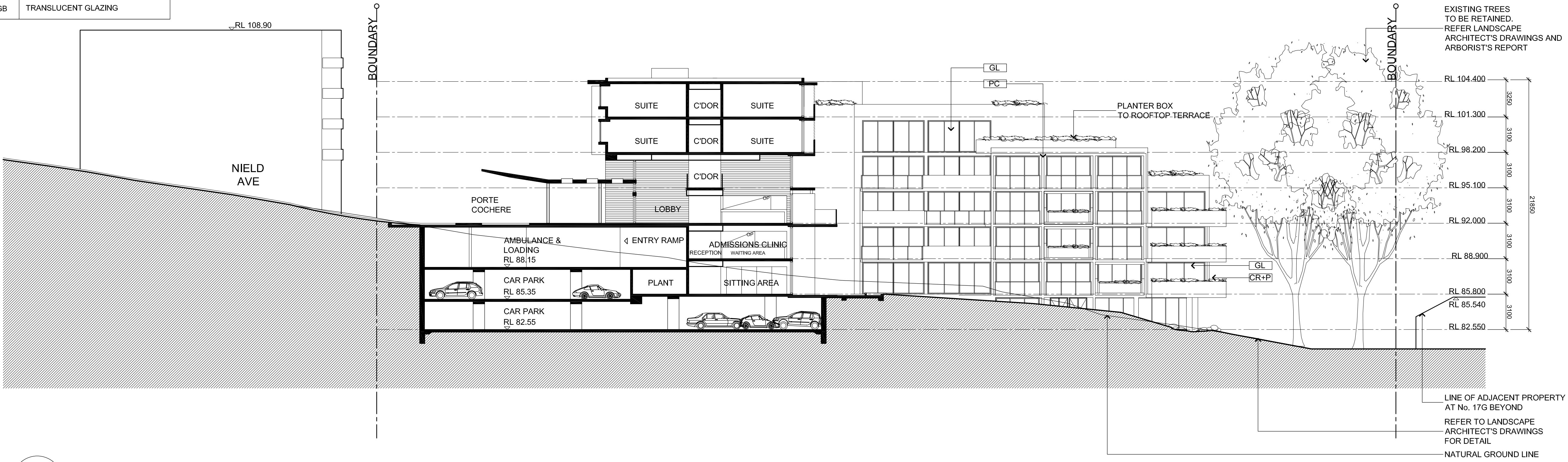
01 SECTION C
