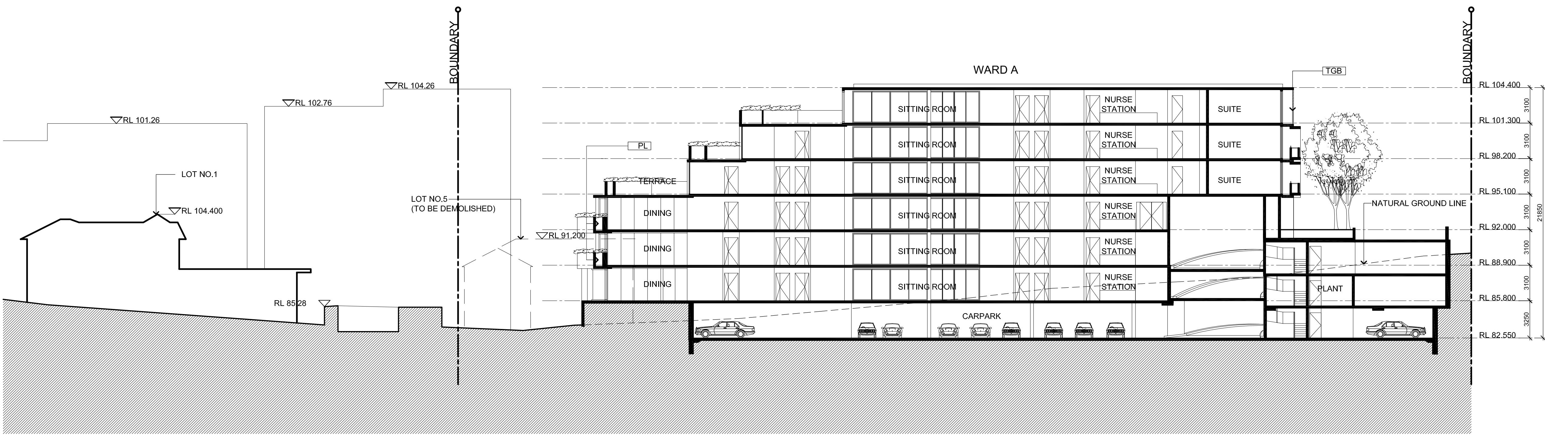
02 SECTION D
