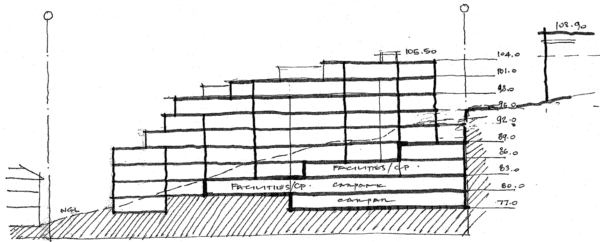
SECTION A-A.
