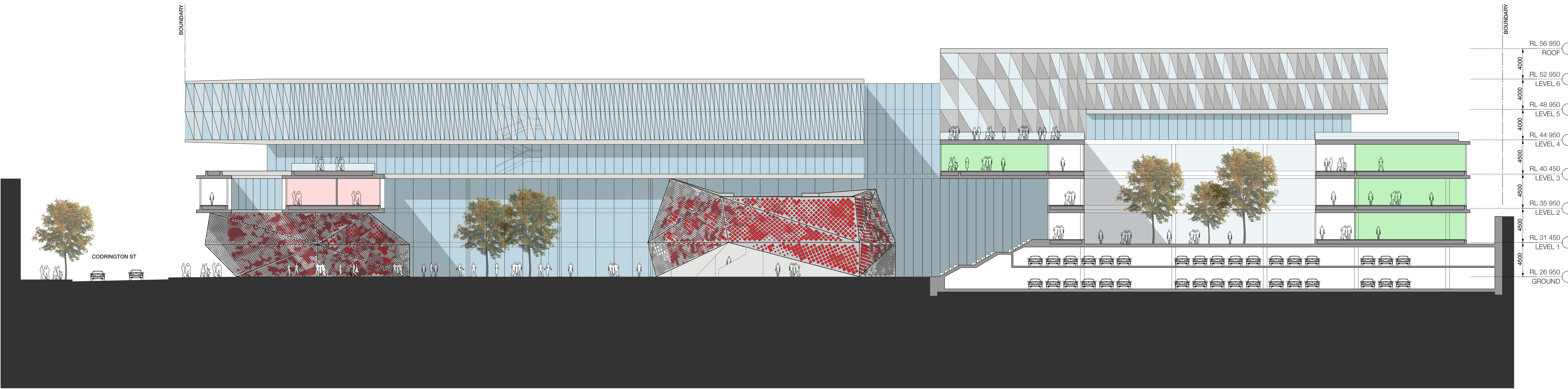
01 SECTION E 1:250 @ A1
