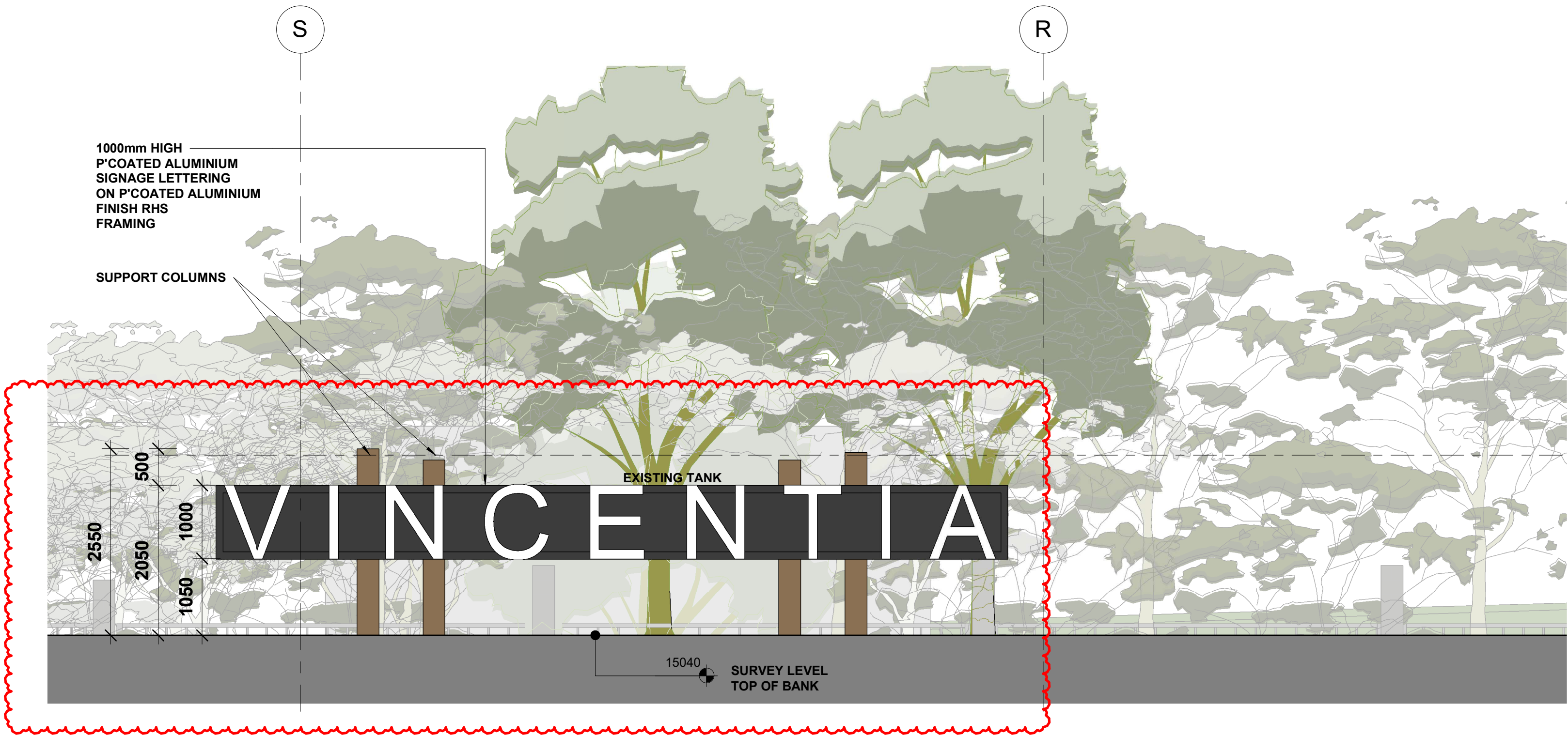
1 OPTION 01 - SIGNAGE TYPE - A 1 : 50
