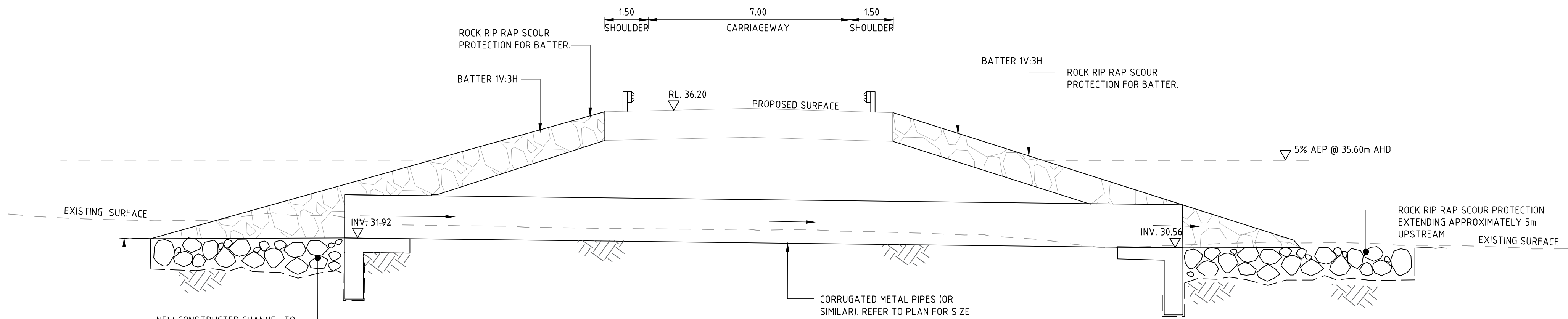
CHAINAGE 612 CULVERT
