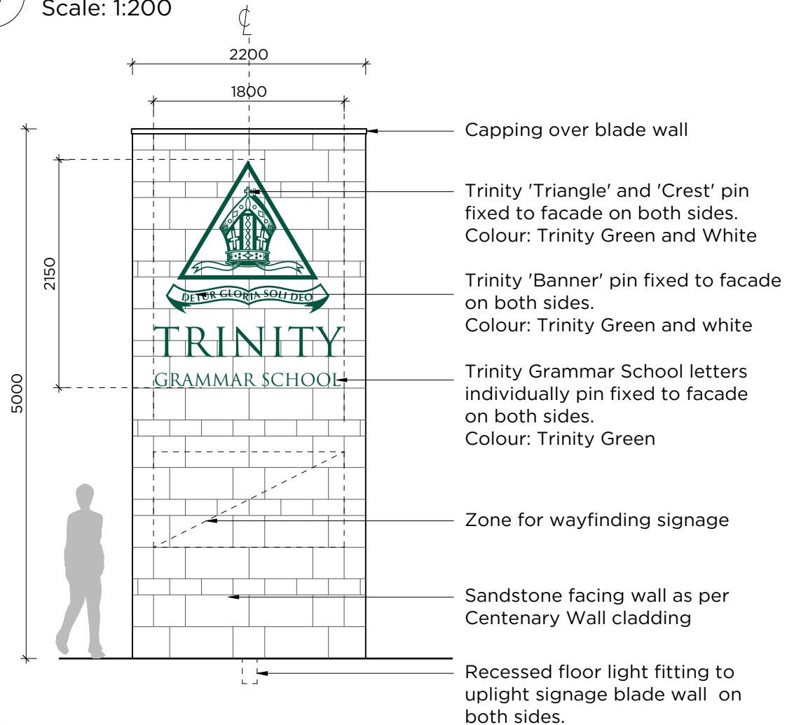
03 Signage Blade Wall Scale: 1:50
