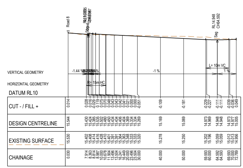
Lane 4 LONGITUDINAL SECTION Scales: HORZ 1 : 500 VERT 1 : 100
