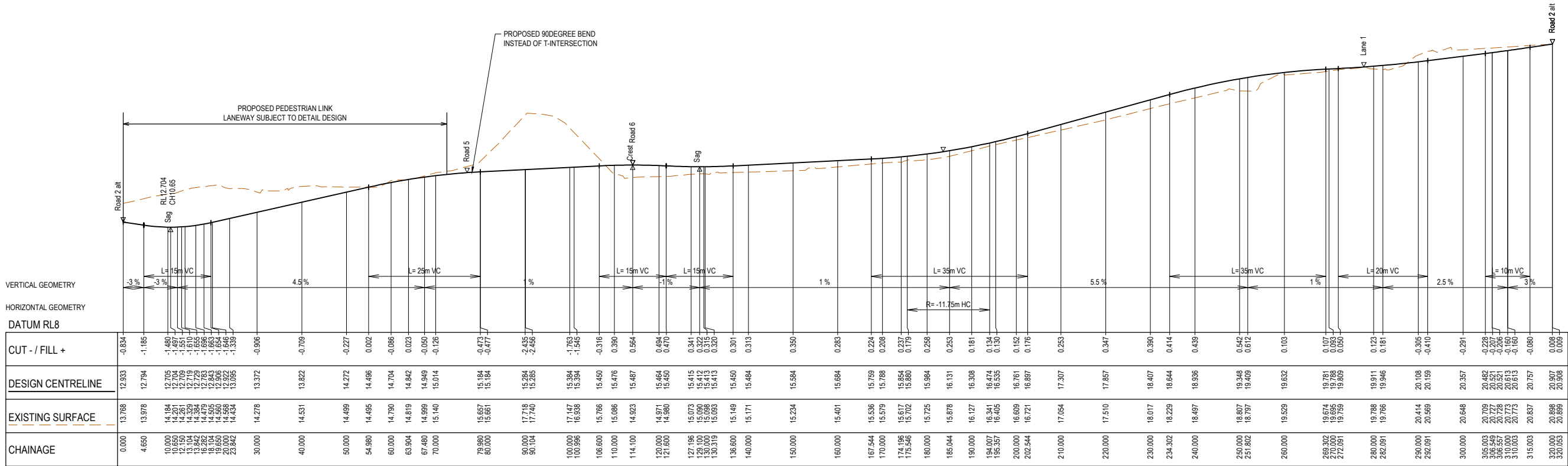
Road 3 LONGITUDINAL SECTION Scales: HORZ 1 : 500 VERT 1 : 100
