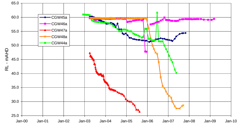
Piezometers CGW44a, 45a, 46a, 47a, 48a - Permian
