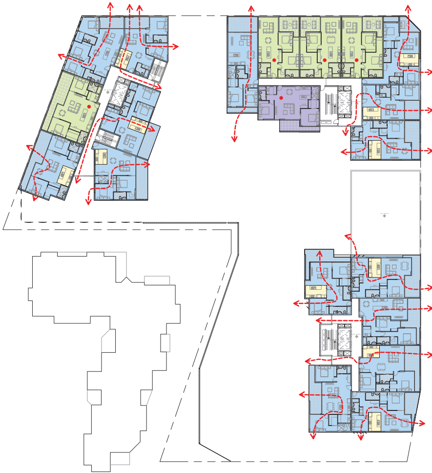
② LEVEL 4 1 : 250
