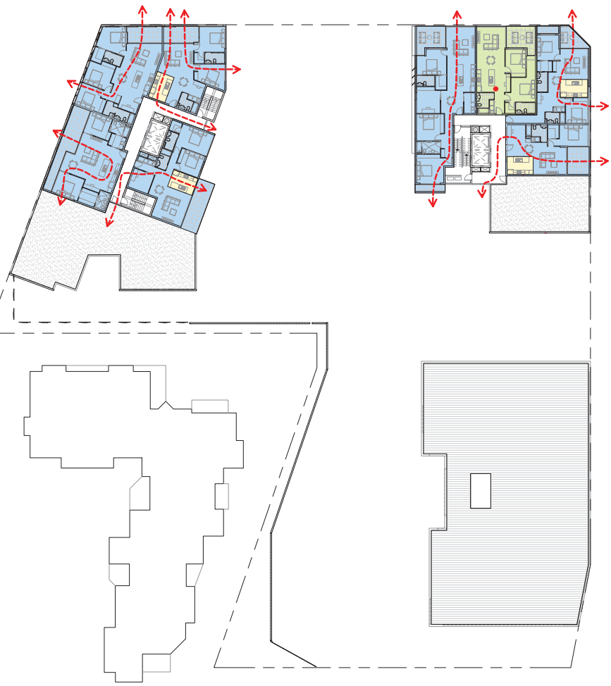
① LEVEL 10 - 15 1:250
