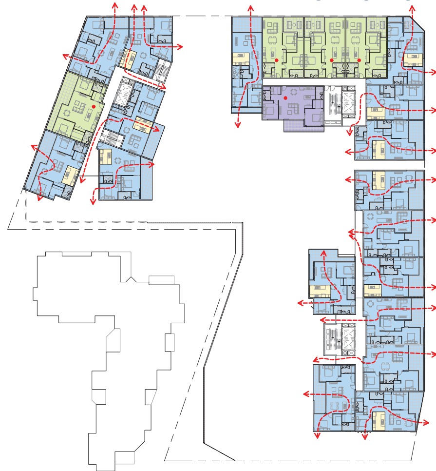
② LEVEL 3 1 : 250
