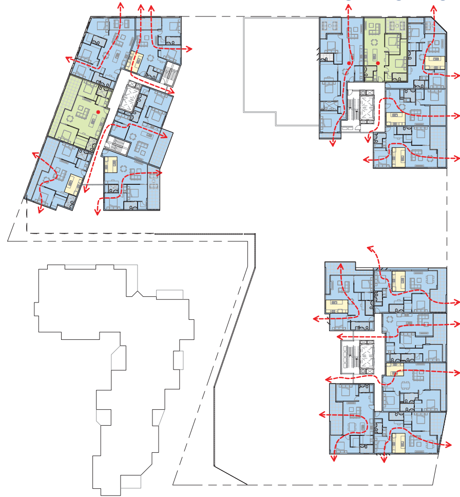
① LEVEL 5 - 9 1 : 250
